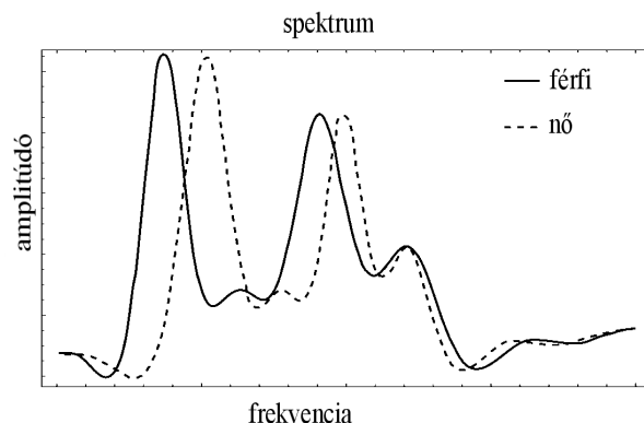
4. ábra Az artikulációs csatorna hosszának frekvenciaeltoló hatása. A képen egy férfi és egy nő által bementett magánhangzó spektruma látható egy adott pillanatban.
